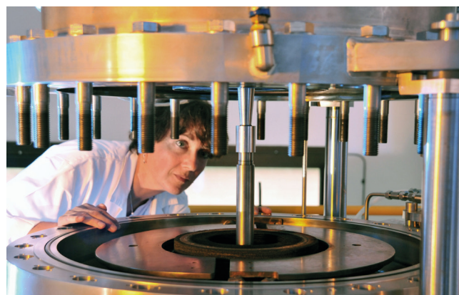
Four bridgman pour l'élaboration de céramiques
